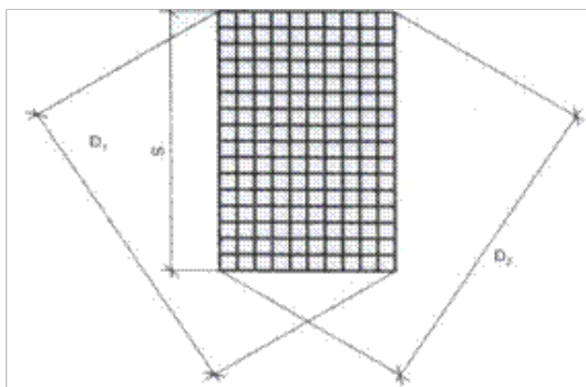
Verschil van de diagonaalmaten D1 minus D2 max. 0,12 x S
