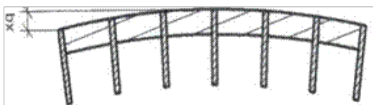
Bolrond bx max. 1/150 van de breedte >450mm; max. 8mm; <450mm max. 3mm
