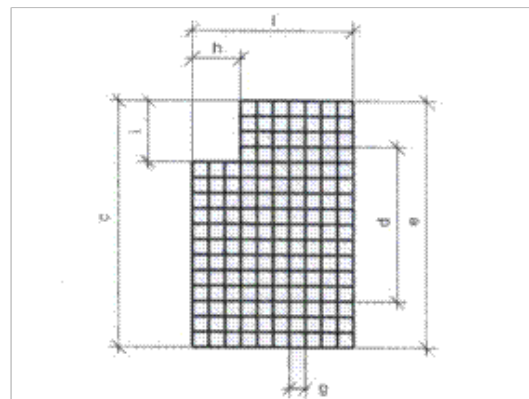
c; e; f = max. +0 tot -4mm; g = max. \pm 1,5 \text{ mm} ; d = max. +4 tot -4mm (over 10 delingen); h; i = +8 tot -0mm
