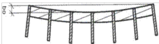
Holrond bo max. 1/200 van de breedte >600mm;
